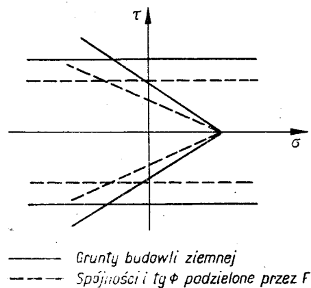
Rys. 7. Współczynnik wytrzymałości całkowitej
